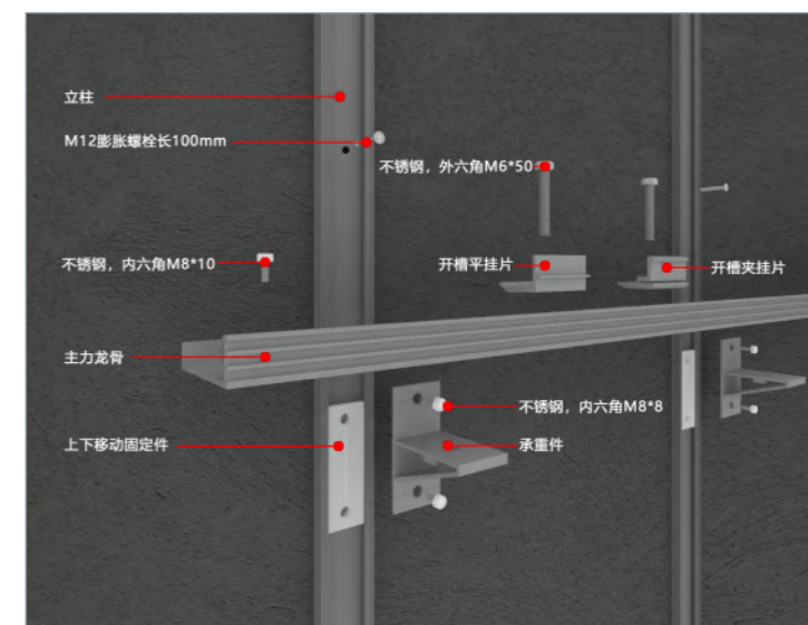
9平方米背景墙悬空龙骨配置表
