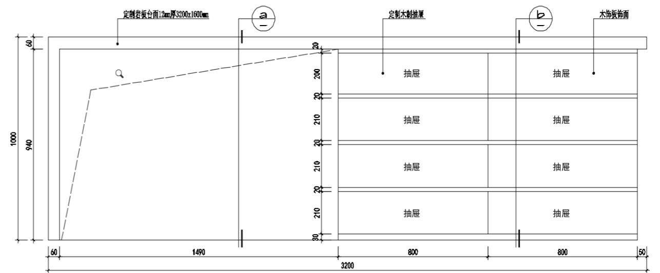
结构图
