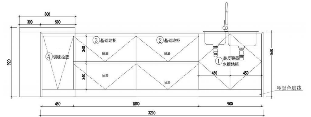
结构图
