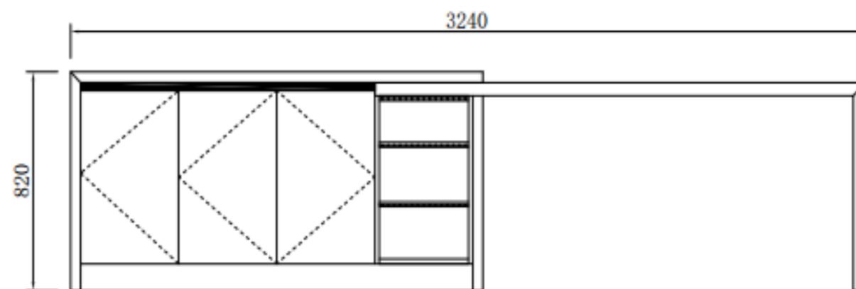
结构图
