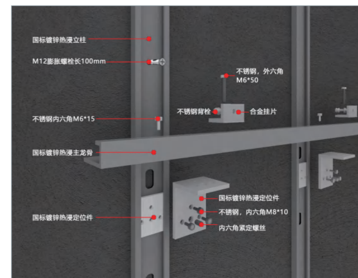
9平方米外墙干挂镀锌龙骨配置
